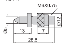
测砧
